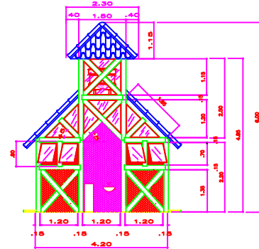
FACHADA PRINCIPAL / ESC. 1:50 GEOMETRICO
