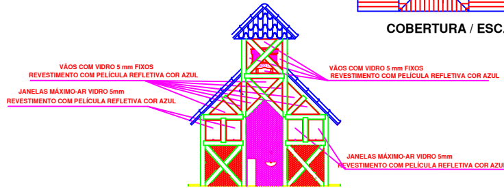
FACHADA FRONTAL / ESC. 1:50
