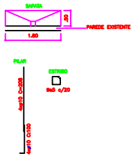
DET. PILAR DE CONCRETO
