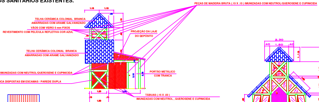
VISTA LATERAL / ESC. 1:50
