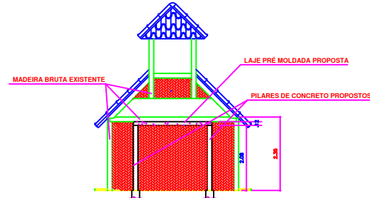
CORTE LONGITUDINAL AB ESC. 1:50
